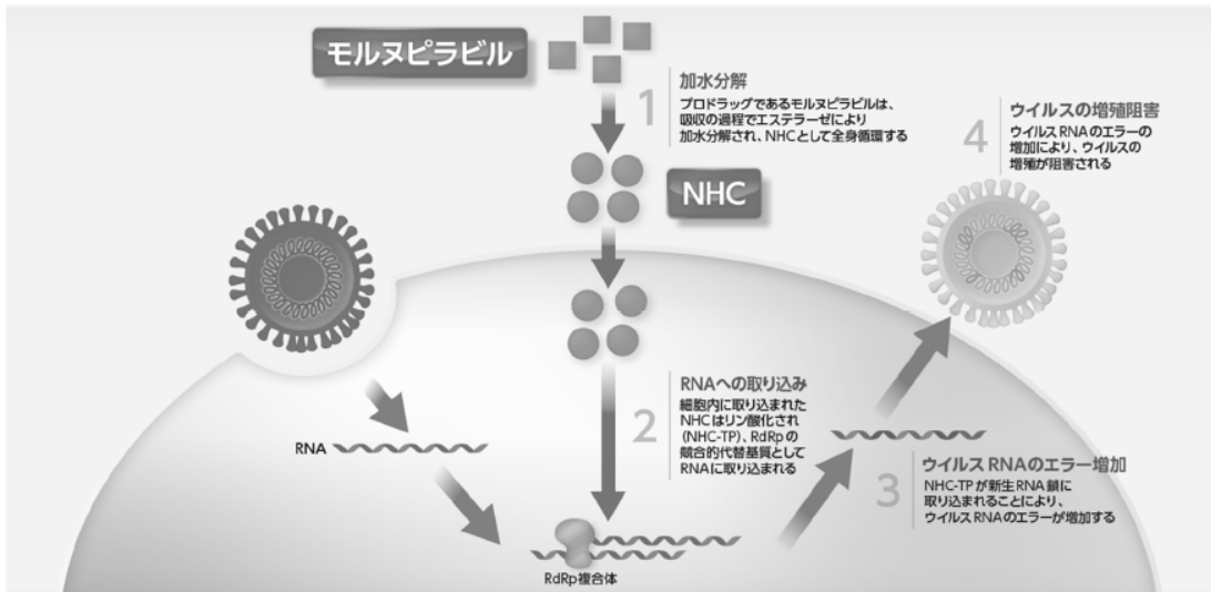
モルヌピラビルの作用機序
